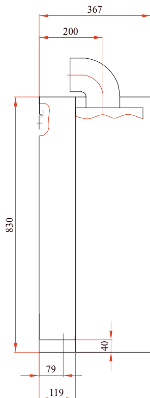
ŘEZ I-I
