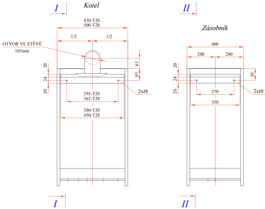
ŘEZ I-I
